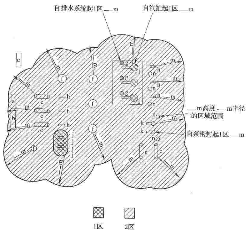
(a) 平面图
