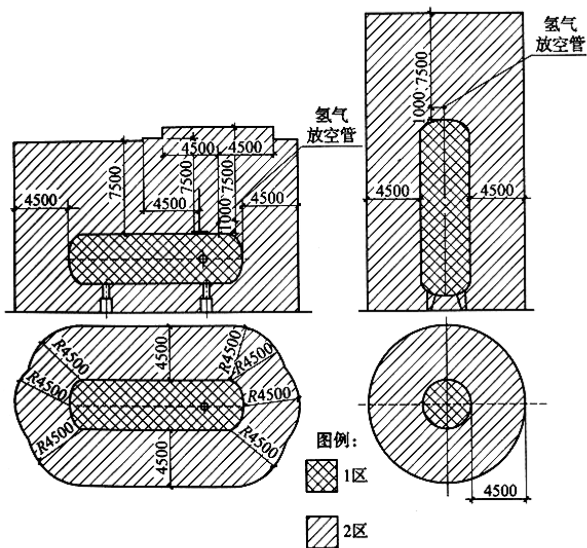
图 A.0.3 氢气站内的室外制氢设备、氢气罐爆炸危险区域划分
