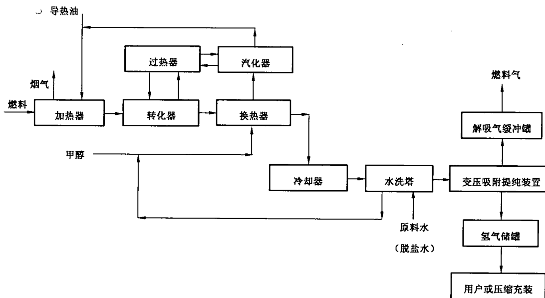
图 A.3 甲醇转化制氢系统框图
